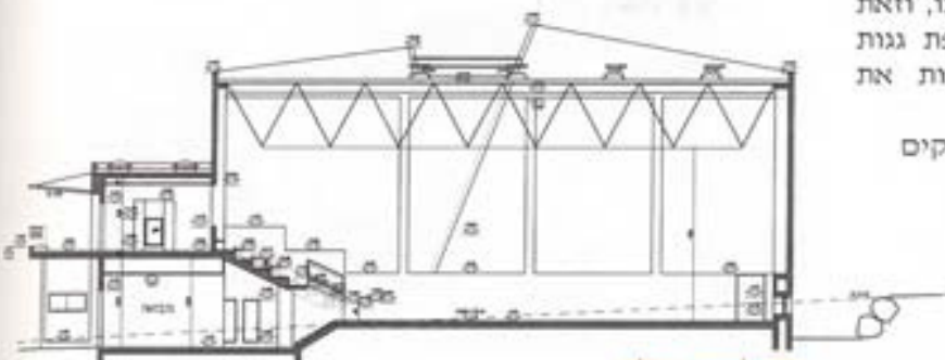
חתך לרוחב האולם
